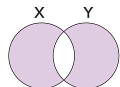
図4: 排他的論理和 ベン図 着色部分
